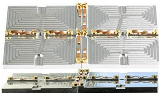
EM-Tec G4.0 地質薄片ホルダー 岩石スライド 4 枚用 最大 28×48mm、M4
