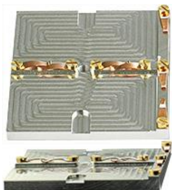
EM-Tec G2.0 地質薄片ホルダー 最大 28×48mm の岩石スライド 2 枚用、M4
